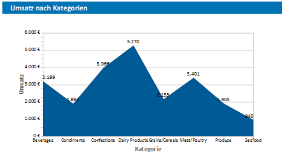
Abbildung 6.15: Gestapeltes Flächendiagramm
