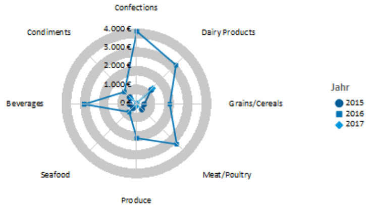
Abbildung 6.23: Gestaffeltes Netzdiagramm
