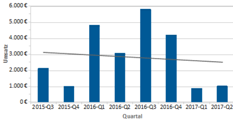
Abbildung 6.31: Ausgleichsgerade
