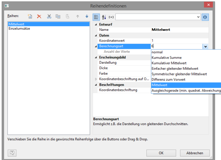
Abbildung 6.30: Reihendefinition
