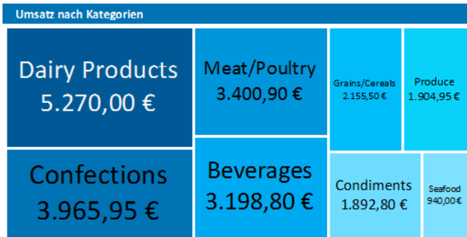
Abbildung 6.24: Treemap
