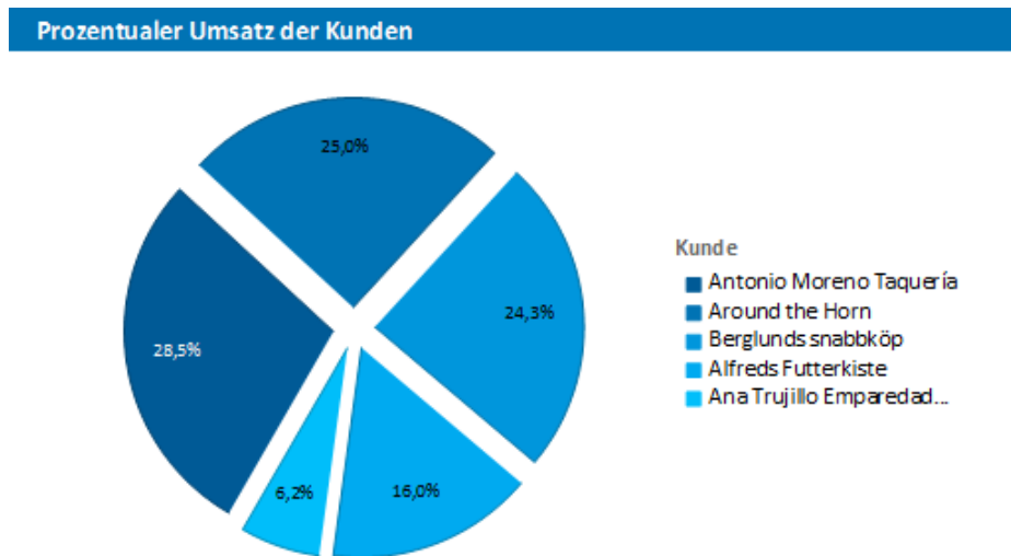
Abbildung 6.4: Kreisdiagramm
