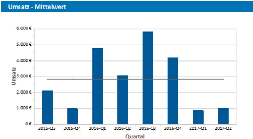
Abbildung 6.28: Mittelwertgerade
