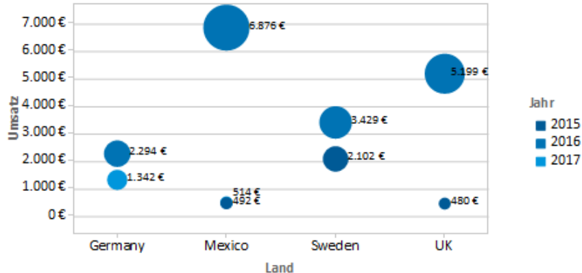
Abbildung 6.16: Verteiltes Blasendiagramm
