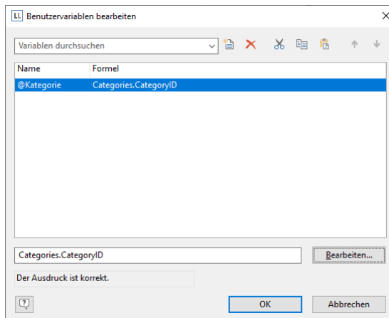
Abbildung 7.25: Benutzervariablen bearbeiten
