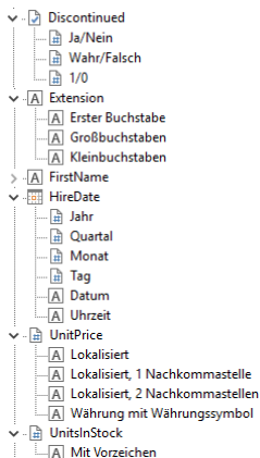
Abbildung 10.2: Virtuelle Formelvariablen
