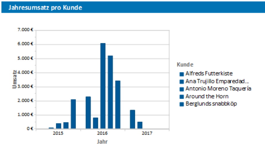
Abbildung 6.8: Gruppirtes Balkendiagramm
