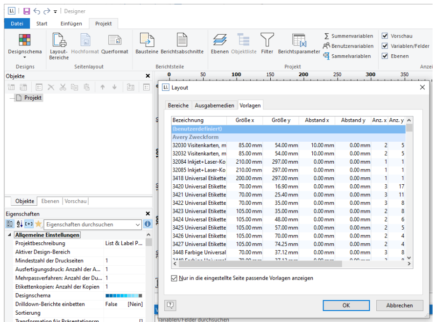
Abbildung 2.65: Etikettenformat festlegen
